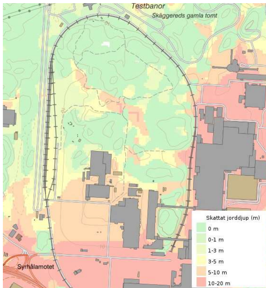
Figur 3 Jorddjupskarta över området (SGU, 2021).
