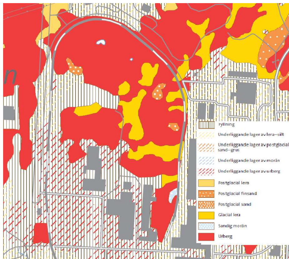
Figur 2 Jordartskarta över området (SGU, 2021).
